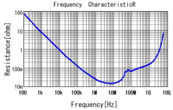
■ GRM188R71H104KA93 R DCOV, 25degC
