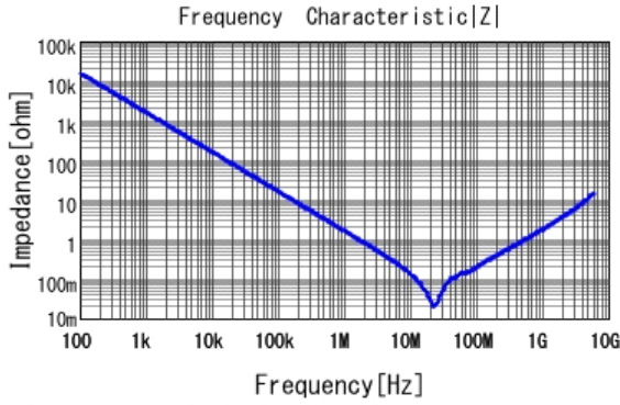
■ GRM188R71H104KA93 |Z| DCOV, 25degC
