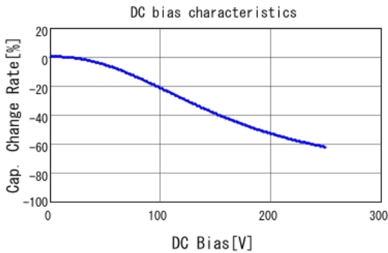
■ GRM188R72E222KW07 C-DC bias capchange, 25.0degC, AC1V
