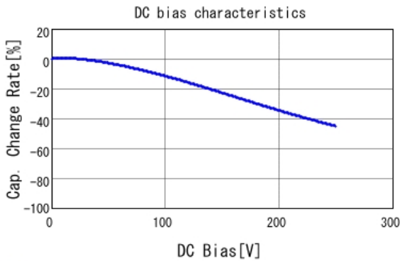
■ GRM188R72E471KW07 C-DC bias capchange, 25.0degC, AC1V
