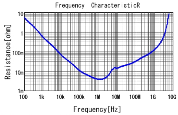
■ GRM219R60J106KE19 R DCOV, 25degC
