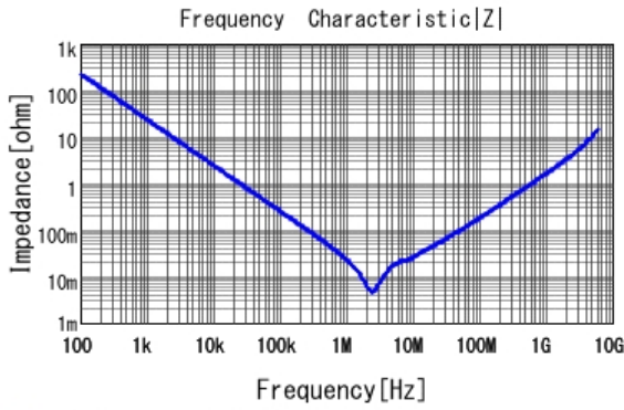
■ GRM219R60J106KE19 |Z| DCOV, 25degC
