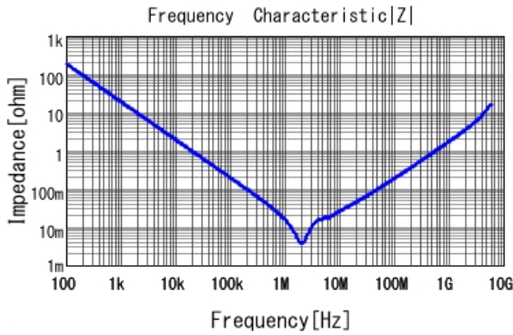
■ GRM21BR60J106KE19 |Z| DCOV, 25degC
