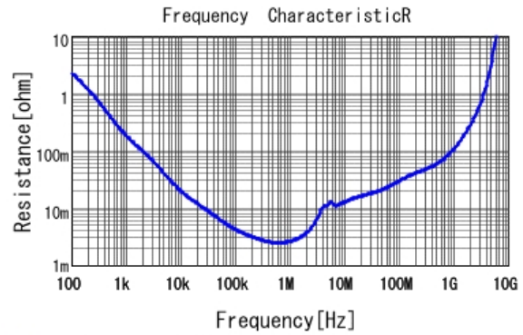
■ GRM21BR60J106KE19 R DCOV, 25degC
