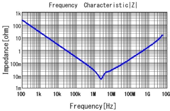
■ GRM21BR70J106KE76 |Z| DCOV, 25degC
