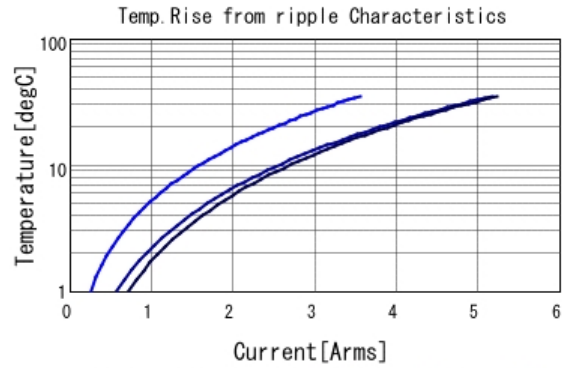
GRM21BR71A106KA73 Temp. rise ■ 80kHz ■ 400kHz ■ 800kHz
