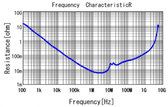
■ GRM21BR71E225KE11 R DCOV, 25degC
