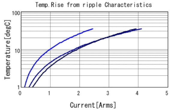
GRM21BR71E225KE11 Temp. rise ■ 100kHz ■ 500kHz ■ 1MHz
