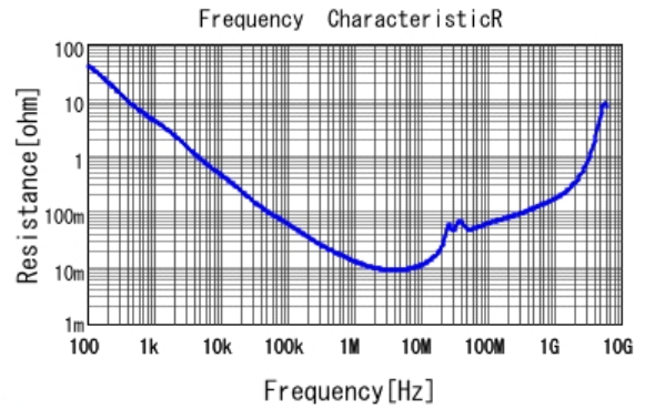
■ GRM21BR71H224KA01 R DCOV, 25degC
