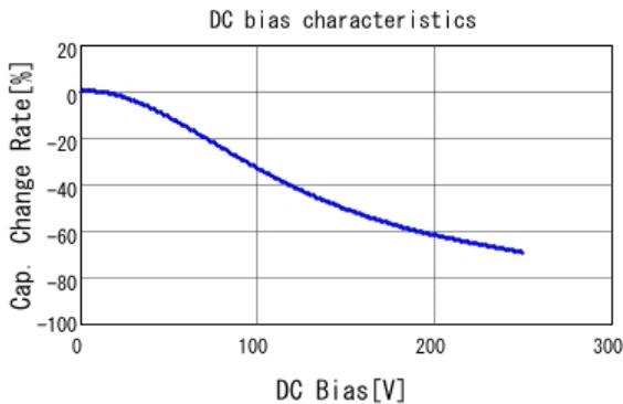
■ GRM21BR72E103KW03 C-DC bias capchange, 25.0degC, AC1V
