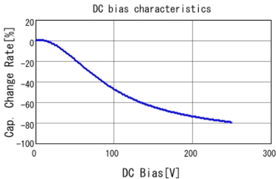
■ GRM21BR72E223KW03 C-DC bias capchange, 25.0degC, AC1V
