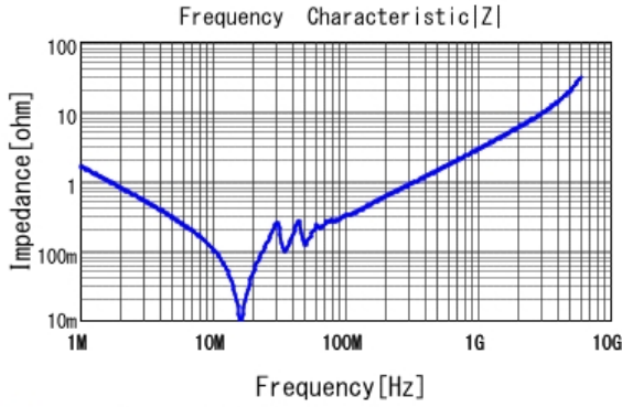
■ GRM31C2C1H104JA01 |Z| DCOV, 20degC
