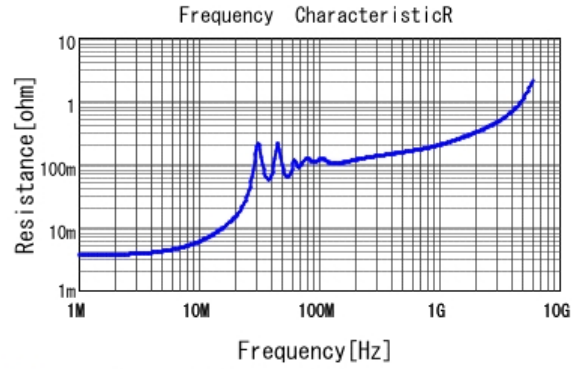
■ GRM31C2C1H104JA01 R DCOV, 20degC
