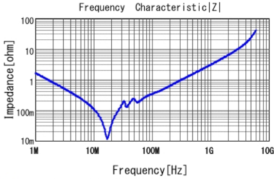
■ GRM31M7U1H104JA01 |Z| DCOV, 25degC
