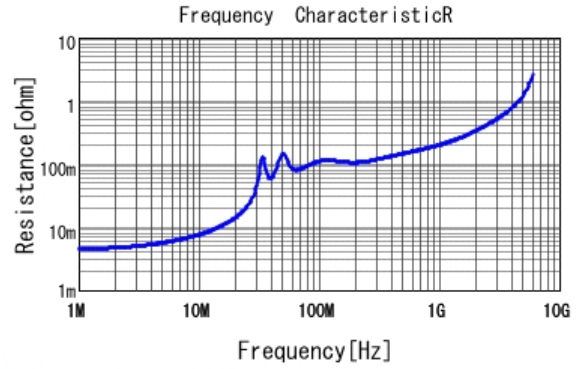
■ GRM31M7U1H104JA01 R DCOV, 25degC
