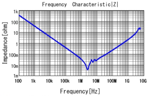
■ GRM32DB11E475KA61 |Z| DCOV, 20degC
