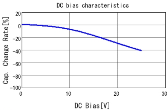
■ GRM32DB11E475KA61 C-DC bias capchange, 20.0degC, AC1.
