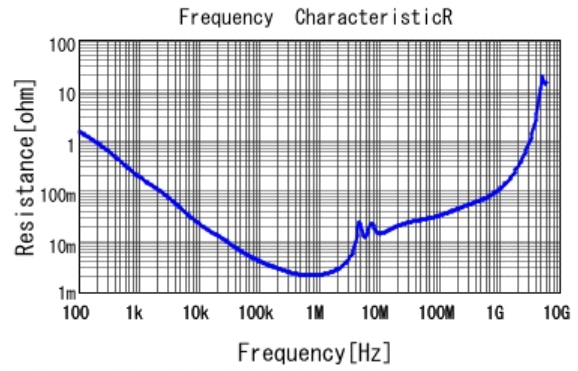
■ GRM32DB11E475KA61 R DCOV, 20degC
