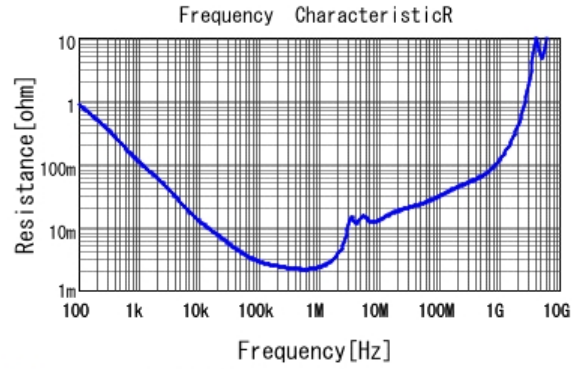
■ GRM32DR71C106KA01 R DCOV, 25degC
