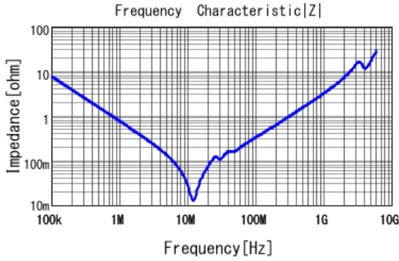
■ GRM32DR72E224KW01 |Z| DC0V, 25degC
