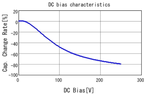
■ GRM32DR72E224KW01 C-DC bias capchange, 25.0degC, AC1V
