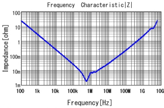
■ GRM32EB30J107ME16 |Z| DCOV, 20degC
