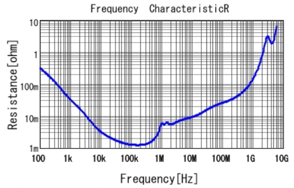
■ GRM32EB30J107ME16 R DCOV, 20degC
