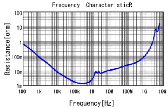
■ GRM32EB31A476KE20 R DCOV, 20degC
