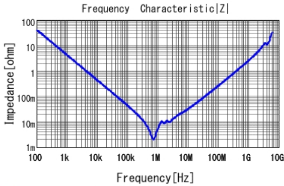
■ GRM32EB31A476ME20 |Z| DCOV, 20degC
