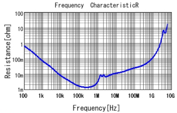
■ GRM32EB31A476ME20 R DCOV, 20degC
