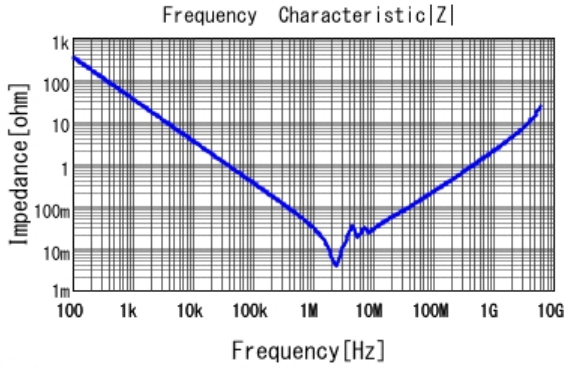
■ GRM32EB31H475KA87 |Z| DCOV, 20degC
