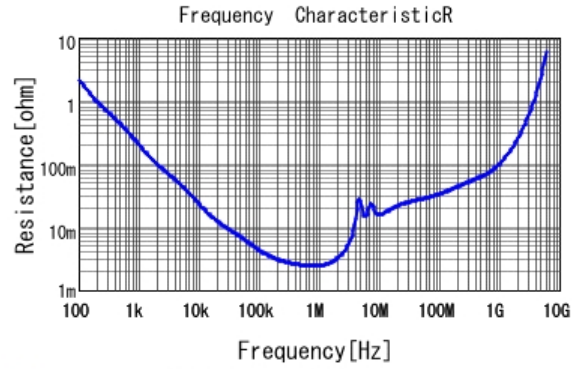
■ GRM32EB31H475KA87 R DCOV, 20degC
