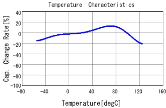
■ GRM32EC70J107ME15 C-Temp. capchange, DCO. 0V, ACO. 18Vr
