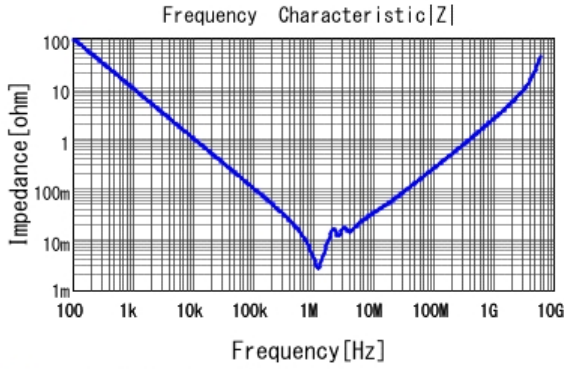
■ GRM32EC81E226KE15 |Z| DCOV, 25degC
