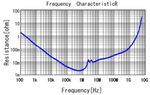
■ GRM32EC81E226KE15 R DCOV, 25degC
