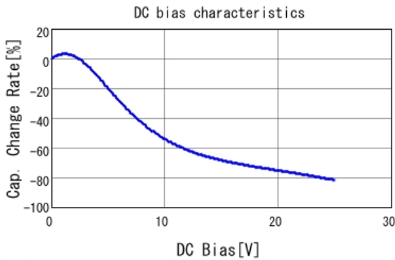
■ GRM32EC81E226KE15 C-DC bias capchange, 25.0degC, AC0.
