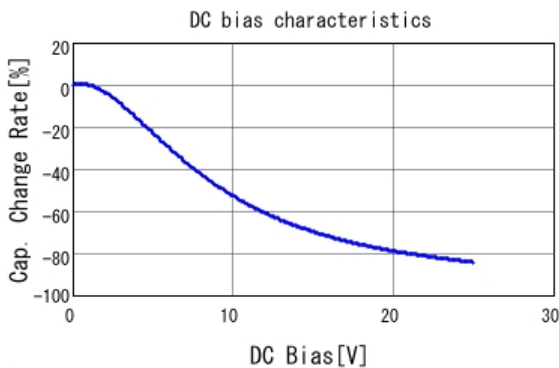
■ GRM32ER61E226KE15 C-DC bias capchange, 25.0degC, AC0.
