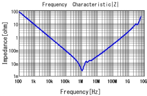
■ GRM32ER61E226KE15 |Z| DCOV, 25degC
