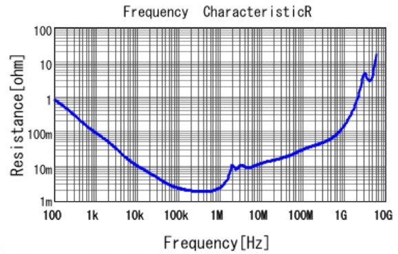
■ GRM32ER61E226KE15 R DCOV, 25degC
