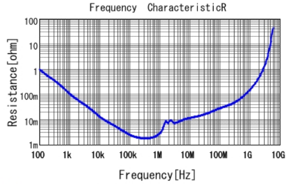
■ GRM32ER71A476KE15 R DCOV, 25degC
