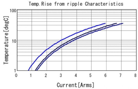
GRM32ER71A476KE15 Temp. rise ■ 60kHz ■ 300kHz ■ 600kHz
