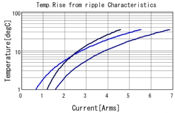
GRM32ER71C226MEA8 Temp. rise ■ 80kHz ■ 400kHz ■ 800kHz
