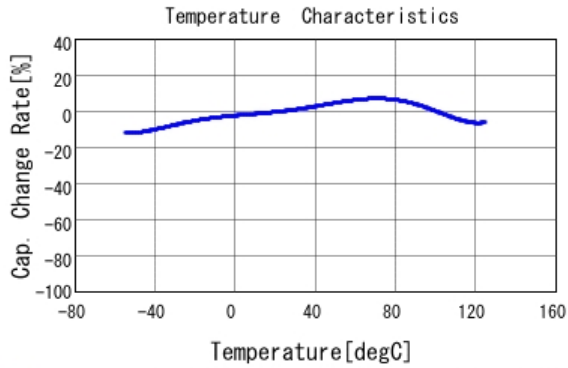
■ GRM32ER71C226MEA8 C-Temp. capchange, DCO. 0V, ACO. 5Vrm
