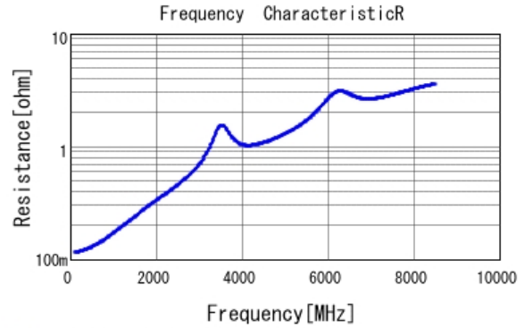
■ GRT1555C1H270JA02 R DCOV, 25degC
