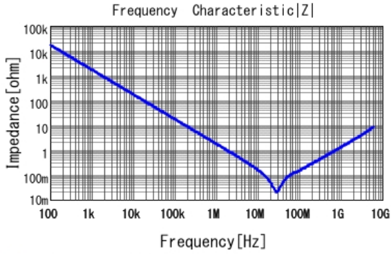
■ GRT155R71H104KE01 |Z| DC0V, 25degC
