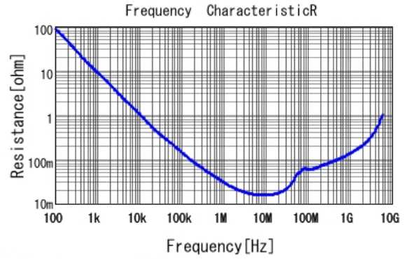
■ GRT155R71H104KE01 R DC0V, 25degC
