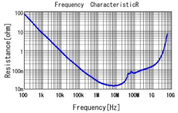
■ GRT188R71H104KE13 R DCOV, 25degC
