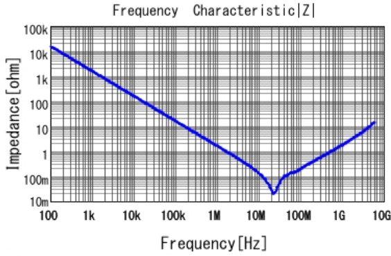
■ GRT188R71H104KE13 |Z| DCOV, 25degC
