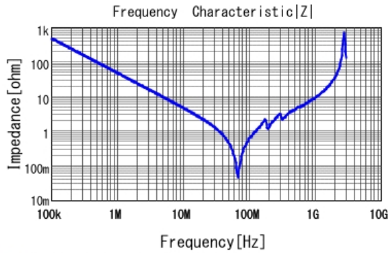
■ KCA55L7UMF332KH01 |Z| DC0V, 25degC
