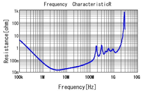
■ KCA55L7UMF332KH01 R DC0V, 25degC
