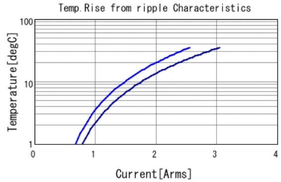
LLL153C70G474ME17 Temp. rise ■ 500kHz ■ 1MHz
