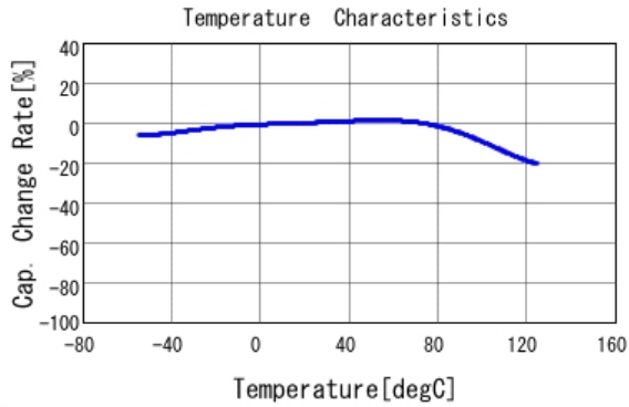
■ LLL153C70G474ME17 C-Temp. capchange, DCO. 0V, ACO. 5Vrm
