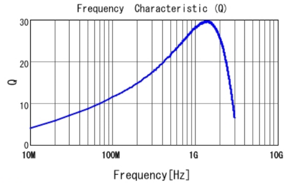
■ LQG15HH12NJ02 Q
