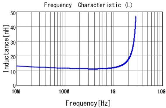
■ LQG15HH12NJ02 L
