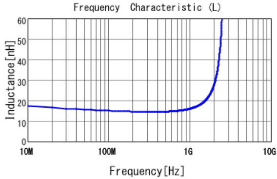
■ LQG15HH15NJ02 L
