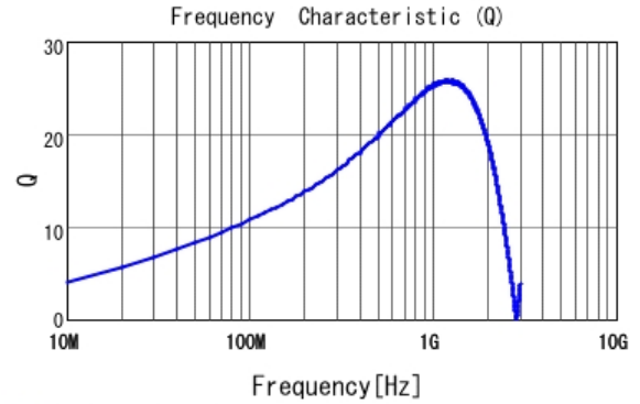
■ LQG15HH15NJ02 Q
