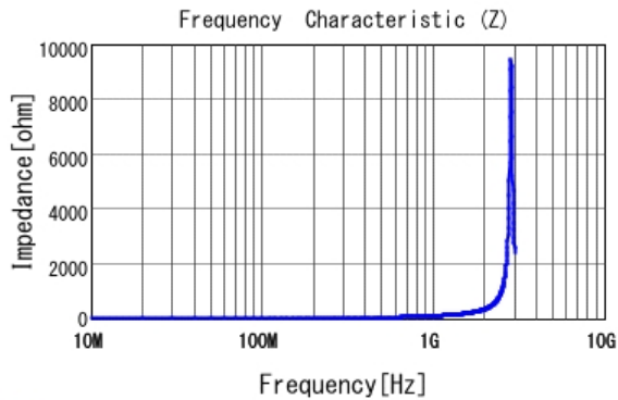
■ LQG15HH15NJ02 |Z|
