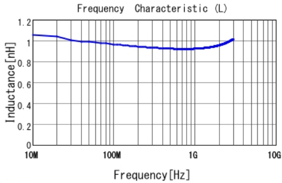
■ LQG15HH1N0S02 L
