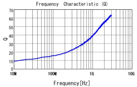
■ LQG15HH1N0S02 Q
