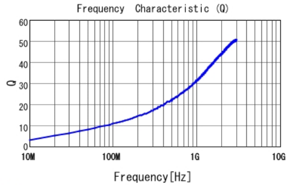
■ LQG15HH2N4S02 Q
