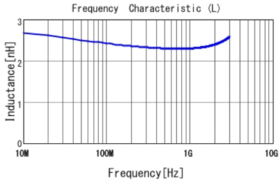
■ LQG15HH2N4S02 L
