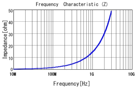
■ LQG15HH2N4S02 |Z|
