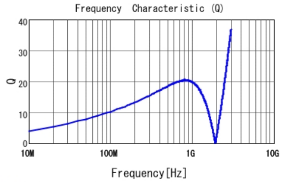
■ LQG15HH33NG02 Q
