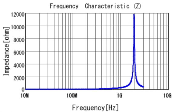
■ LQG15HH33NG02 |Z|
