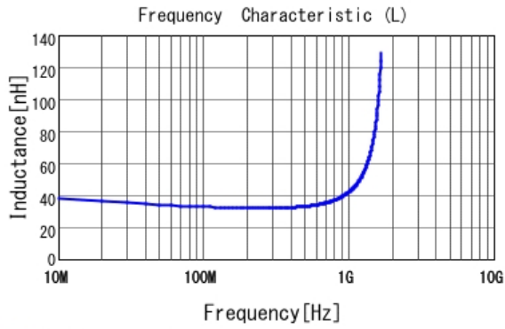
■ LQG15HH33NG02 L
