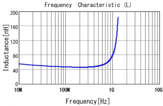
■ LQG15HH47NG02 L
