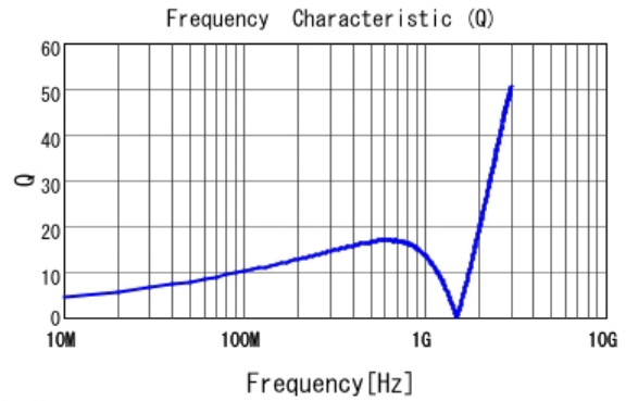
■ LQG15HH47NG02 Q
