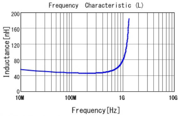
■ LQG15HH47NJ02 L
