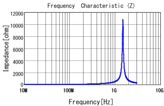
■ LQG15HH47NJ02 |Z|
