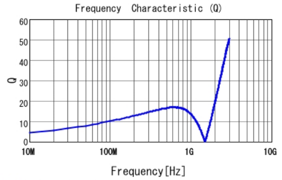
■ LQG15HH47NJ02 Q
