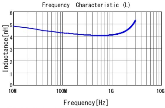
■ LQG15HH4N3S02 L
