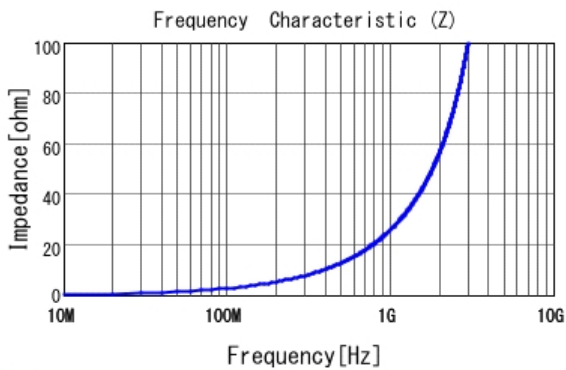
■ LQG15HH4N3S02 |Z|
