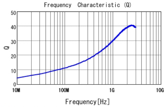
■ LQG15HH4N3S02 Q
