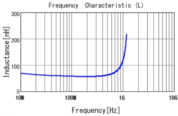
■ LQG15HH56NJ02 L
