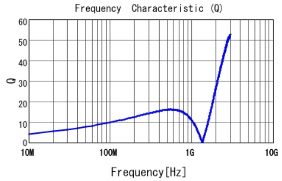
■ LQG15HH56NJ02 Q
