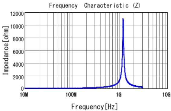
■ LQG15HH68NJ02 |Z|
