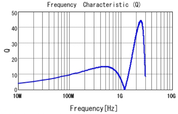
■ LQG15HH68NJ02 Q
