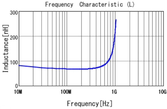
■ LQG15HH68NJ02 L
