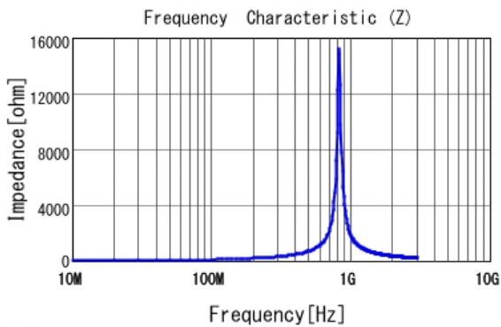
■ LQG15HHR15G02 |Z|
