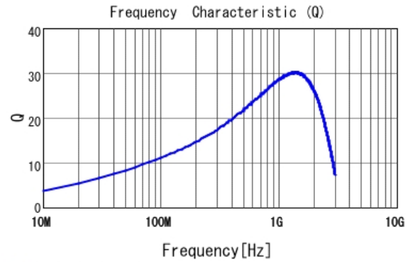
■ LQG15HN12NJ02 Q
