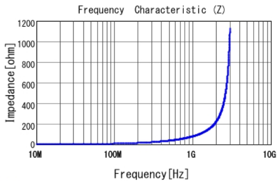
■ LQG15HN12NJ02 |Z|
