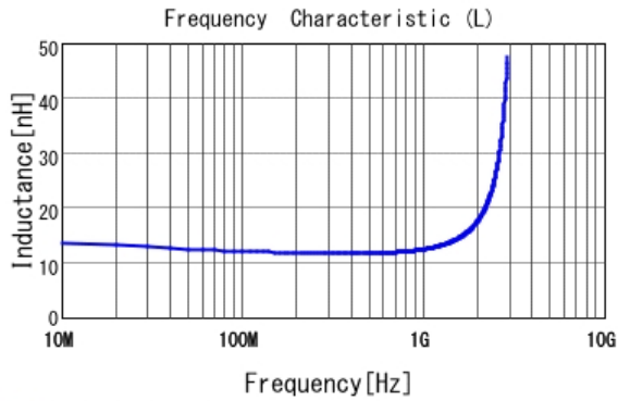
■ LQG15HN12NJ02 L
