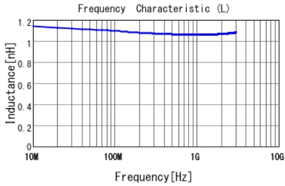
■ LQG15HN1N1S02 L
