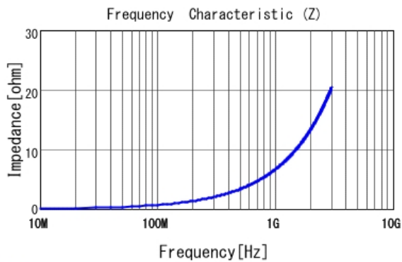
■ LQG15HN1N1S02 |Z|
