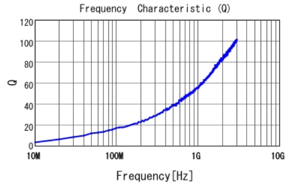
■ LQG15HN1N1S02 Q
