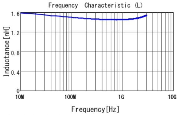
■ LQG15HN1N5S02 L
