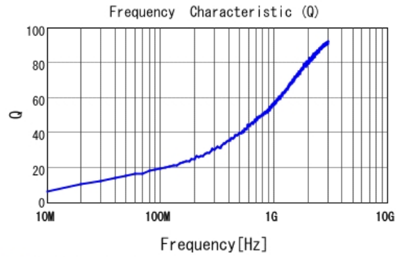
■ LQG15HN1N5S02 Q
