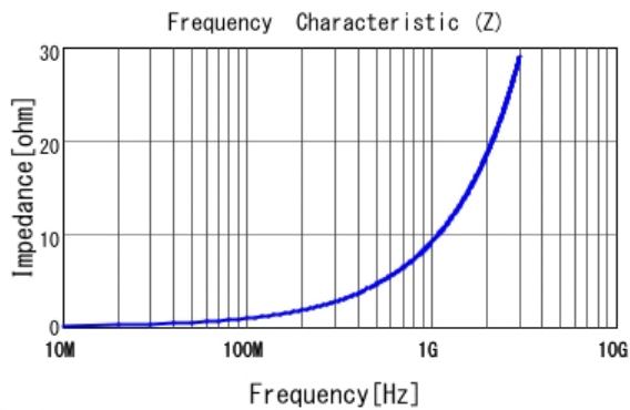
■ LQG15HN1N5S02 |Z|
