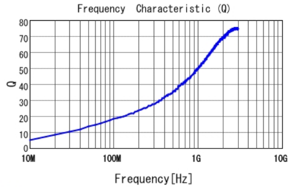
■ LQG15HN1N8S02 Q
