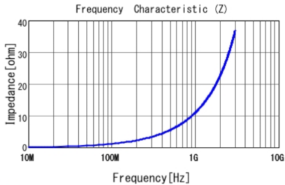
■ LQG15HN1N8S02 |Z|
