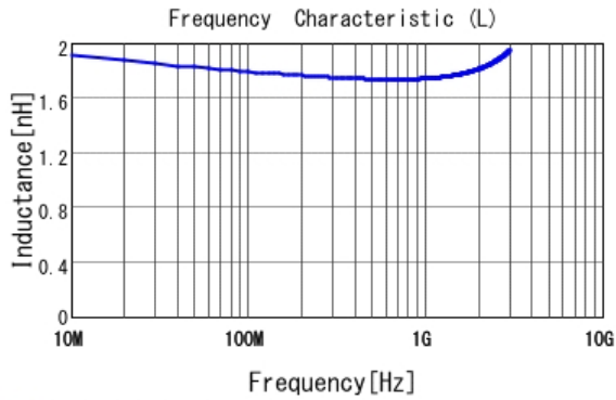
■ LQG15HN1N8S02 L
