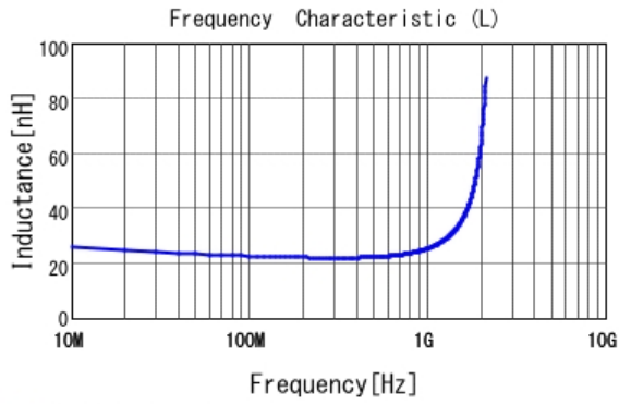
■ LQG15HN22NJ02 L
