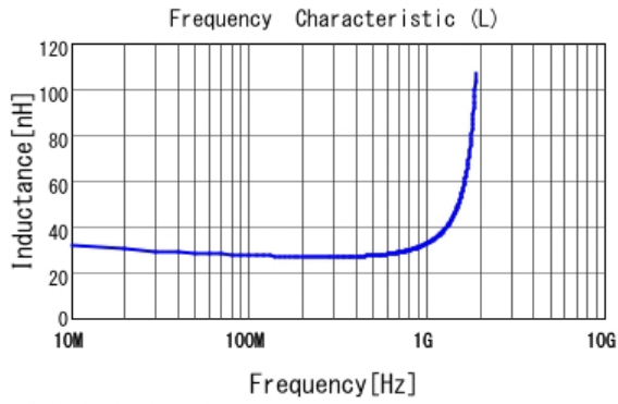
■ LQG15HN27NJ02 L
