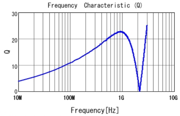
■ LQG15HN27NJ02 Q
