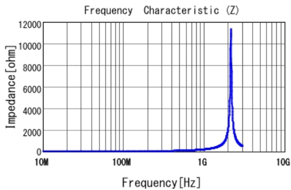
■ LQG15HN27NJ02 |Z|
