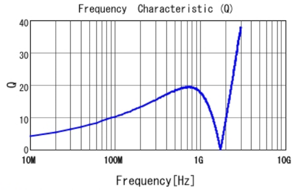
■ LQG15HN39NJ02 Q
