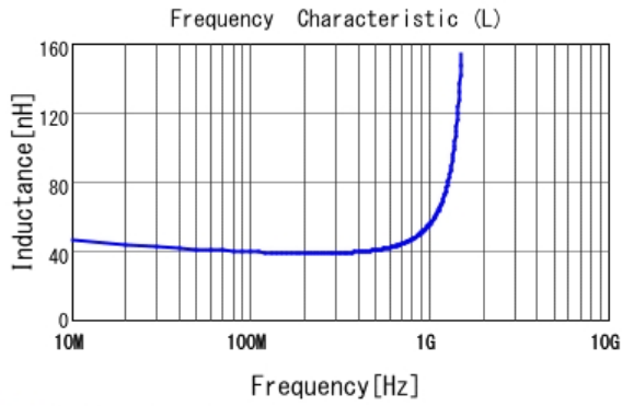
■ LQG15HN39NJ02 L
