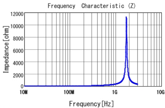
■ LQG15HN39NJ02 |Z|
