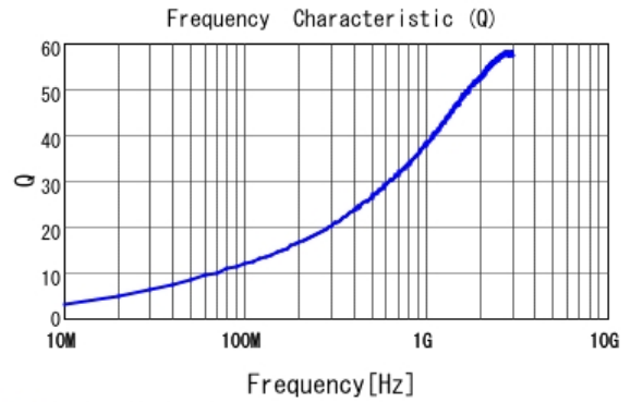
■ LQG15HN3N3S02 Q
