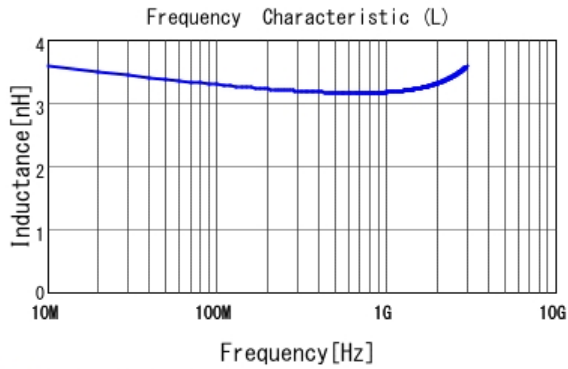
■ LQG15HN3N3S02 L
