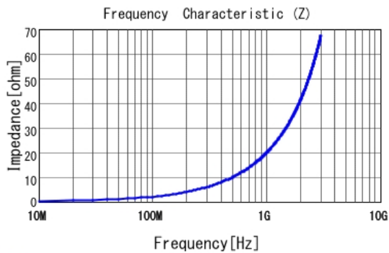
■ LQG15HN3N3S02 |Z|
