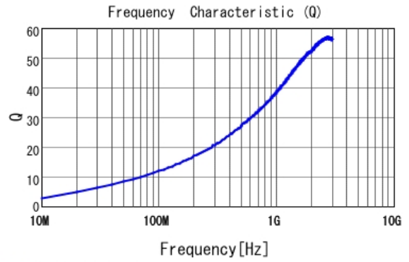
■ LQG15HN3N6S02 Q
