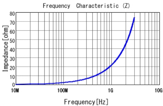
■ LQG15HN3N6S02 |Z|
