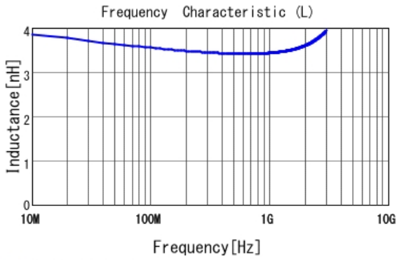
■ LQG15HN3N6S02 L
